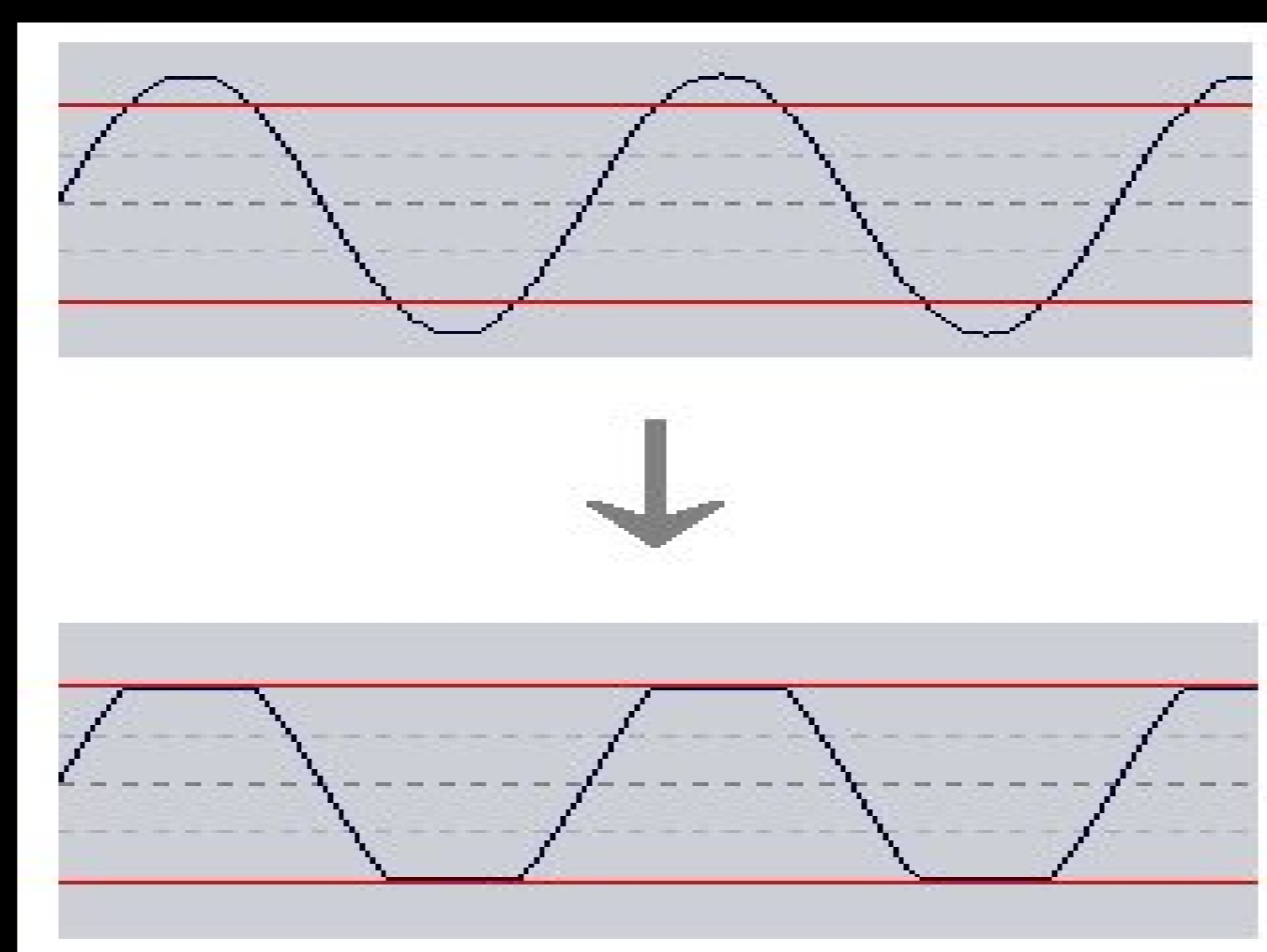
Transformation du signal effectué dans la pédale
