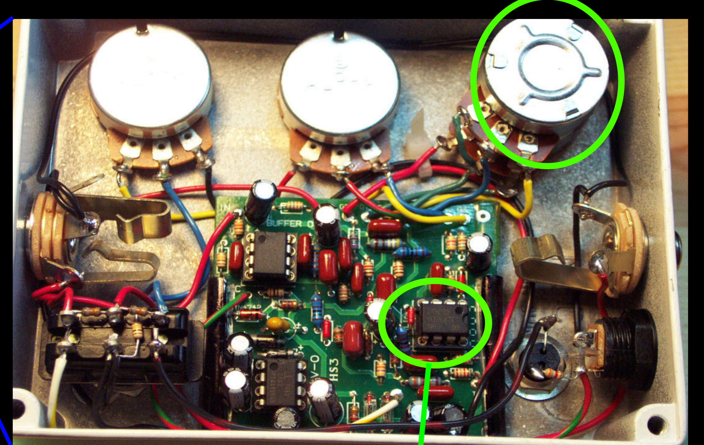
Potentiomètre
