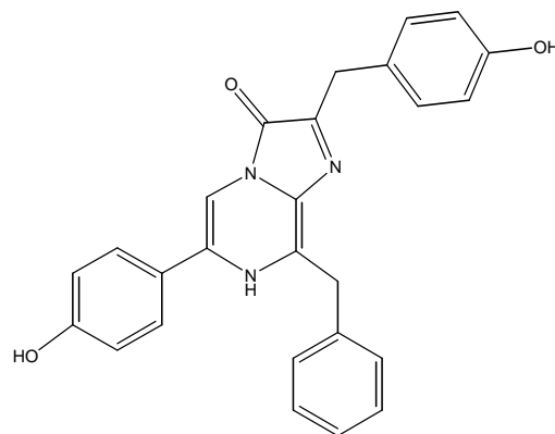
La coelentérazine
