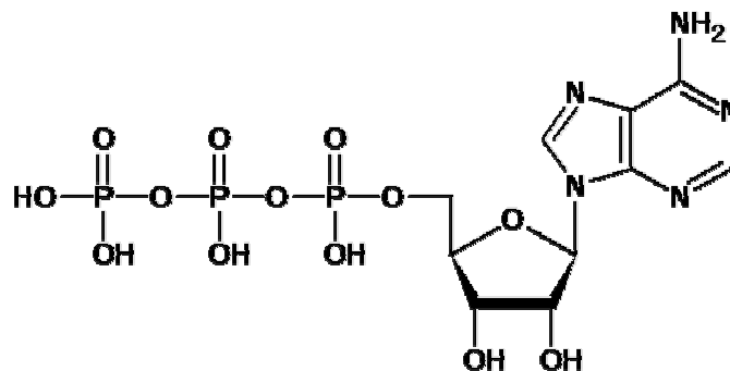
molécule d'ATP
