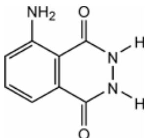
Le luminol
