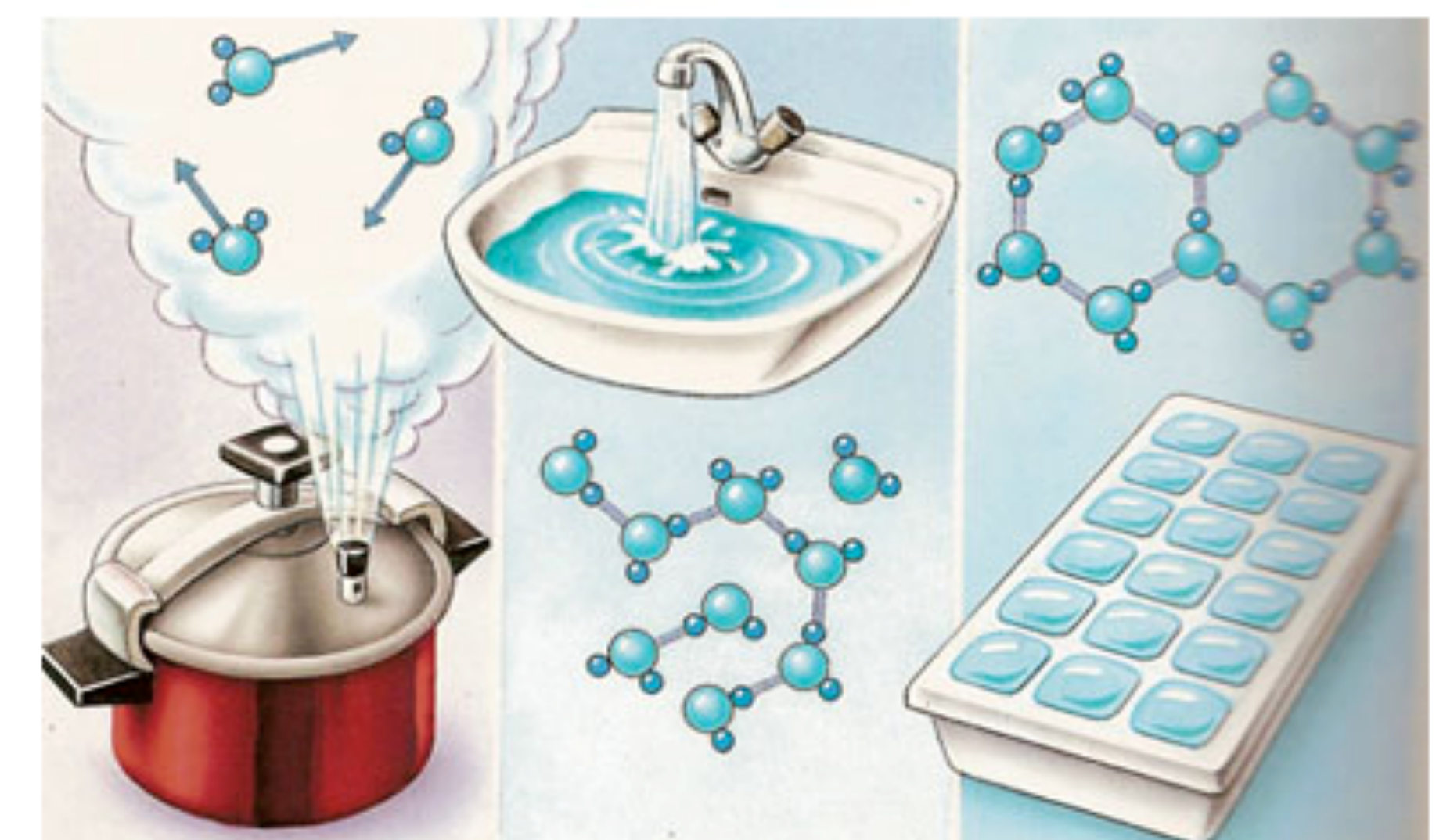
Les liaisons entre molécules d'eau varient en fonction de l'état physique de l'eau.
