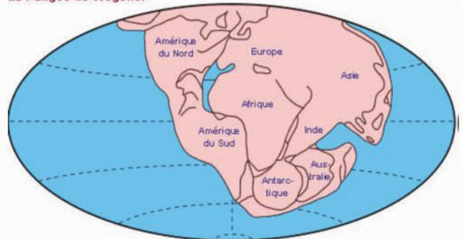
La Pangée de Wegener
