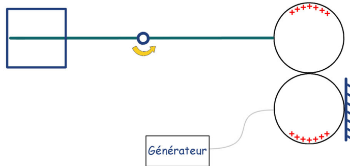
FIG. 1 - Nous chargeons les boules
