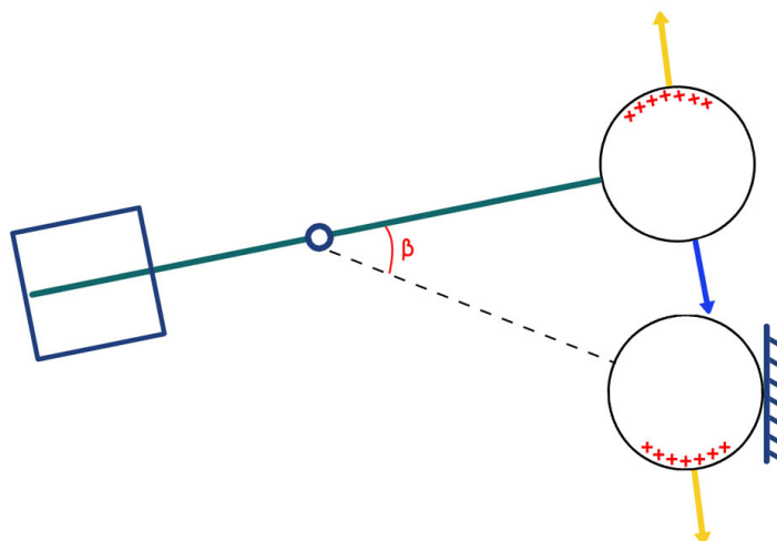
FIG. 3 - Nous tordons le fil pour obtenir une nouvelle force de torsion
