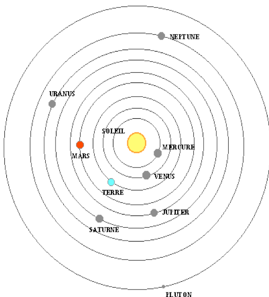
Le Système Solaire et ses Planètes
