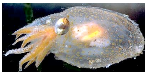
La pieuvre Japetella
