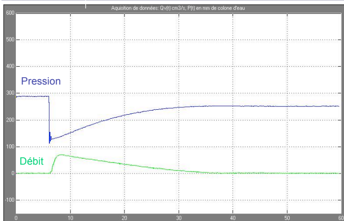
Résultat d'acquisition d'un écoulement non perturbé
